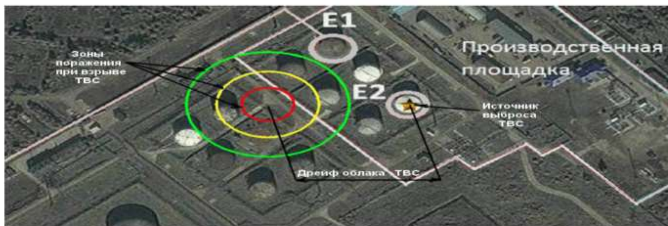
Рис. 1. Зоны поражения ударной волной при взрыве облака ТВС
