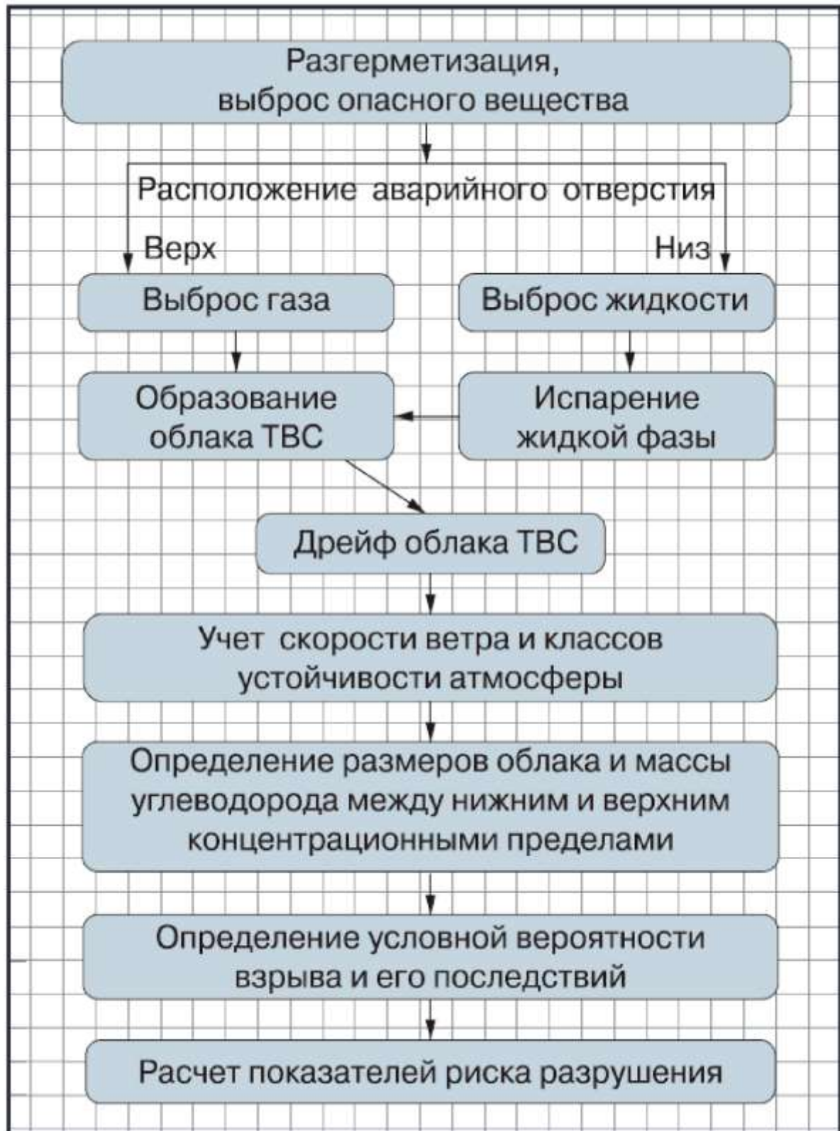
Рис. 2. Алгоритм оценки риска взрыва ТВС
