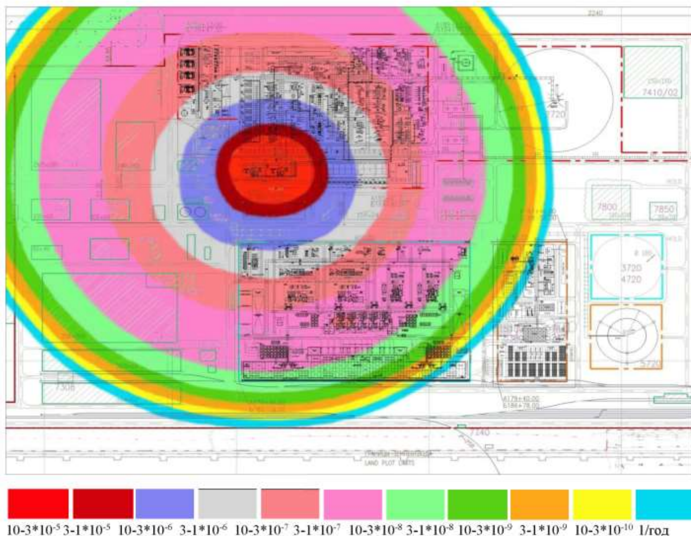
Рис. 5-2. Территориальное распределение потенциального риска разрушения зданий при \Delta P_{\phi} = 12 кПа при авариях на деэтанизаторе со взрывом облака ТВС
