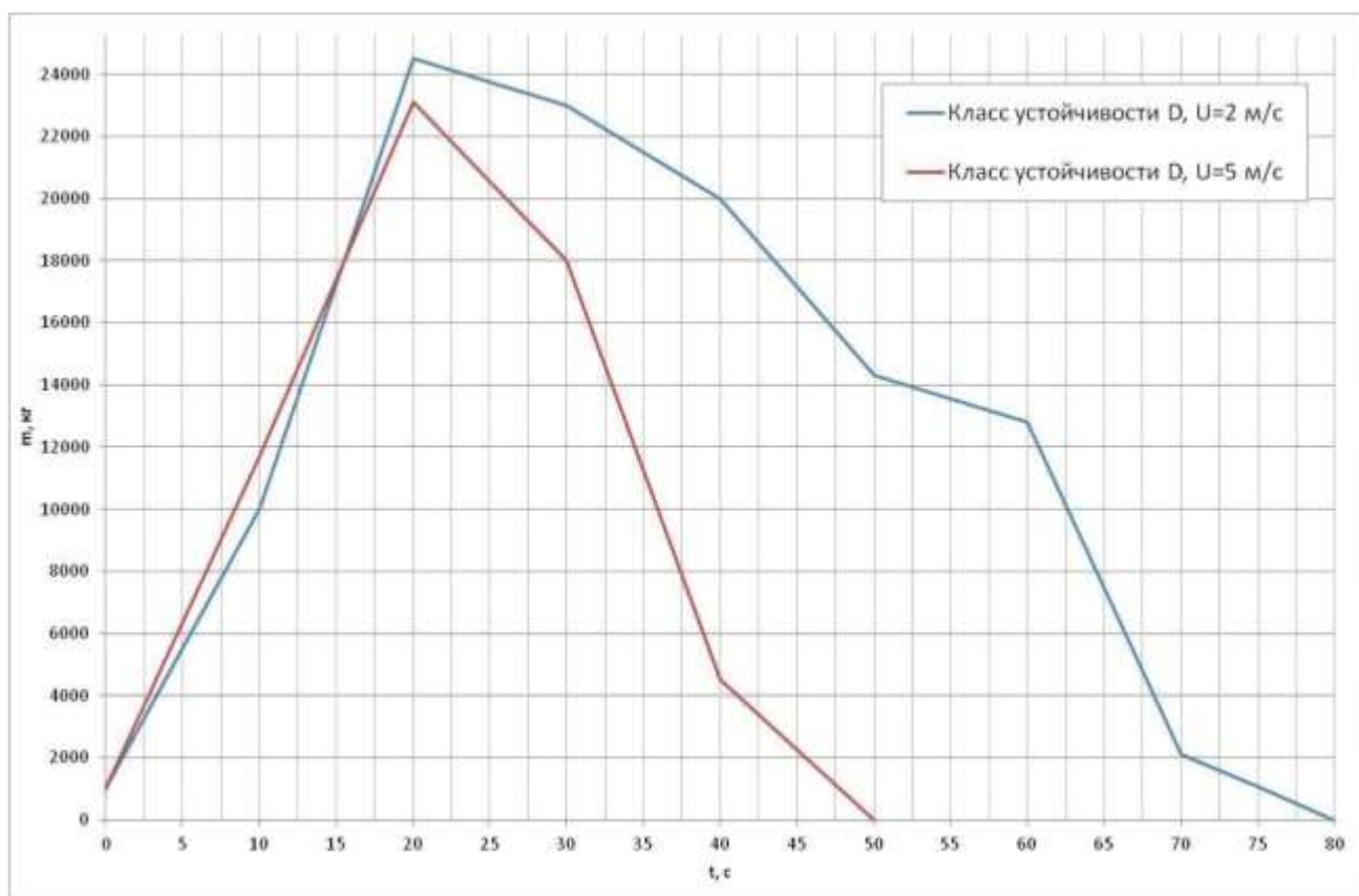
Рис. 5-1. Примеры изменения массы облака M_T при дрейфе в условиях изотермии со скоростями ветра 2 и 5 м/с
