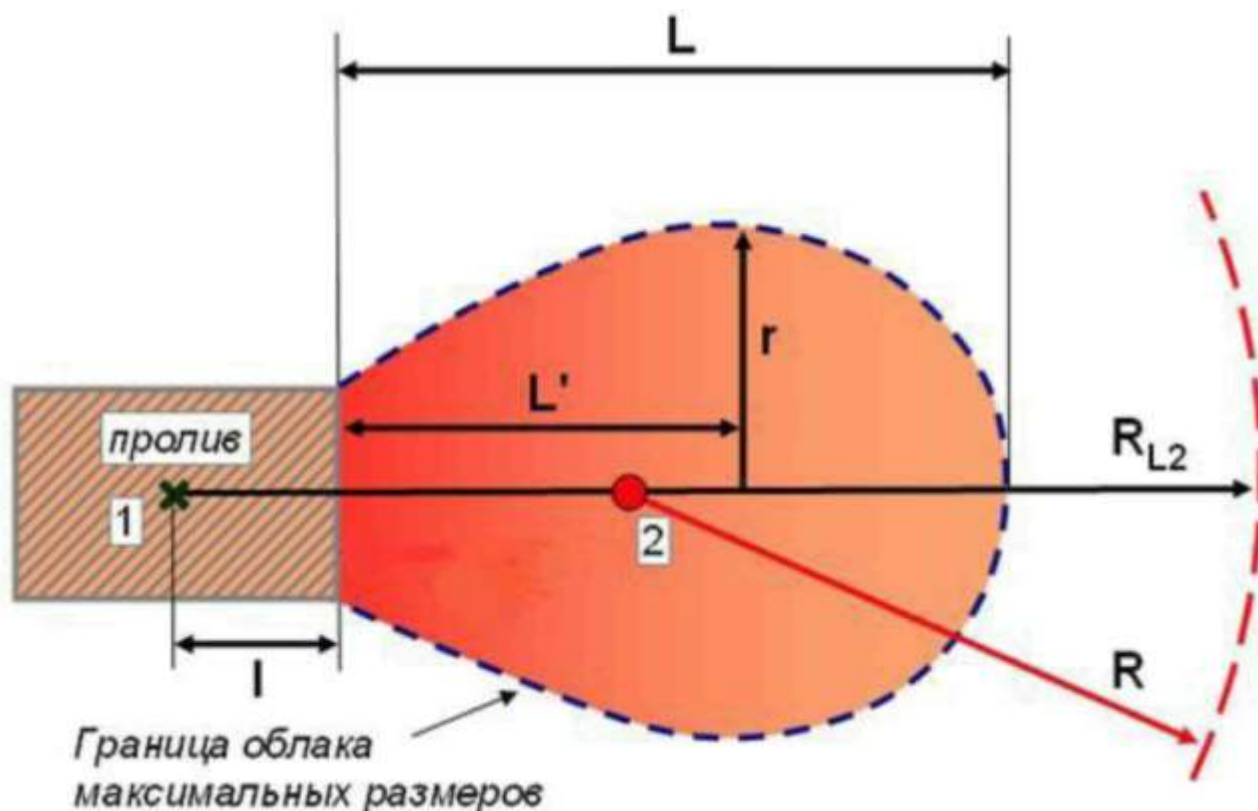
Рис. 4. Схема распространения вторичного облака ТВС при аварийном
