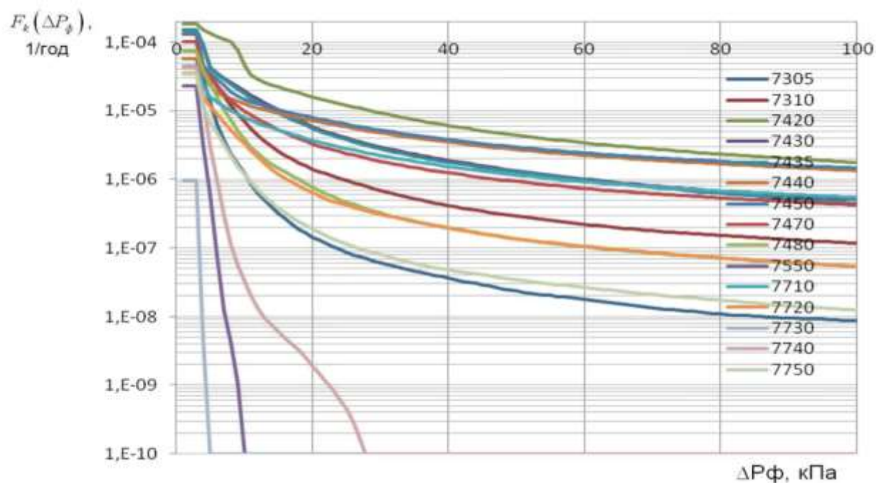
Рис. 5-5. Зависимости частоты F_k превышения избыточного давления \Delta P_{\phi} на
